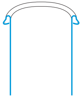
FLARED RIM SCHRÄGER ROLLRAND
